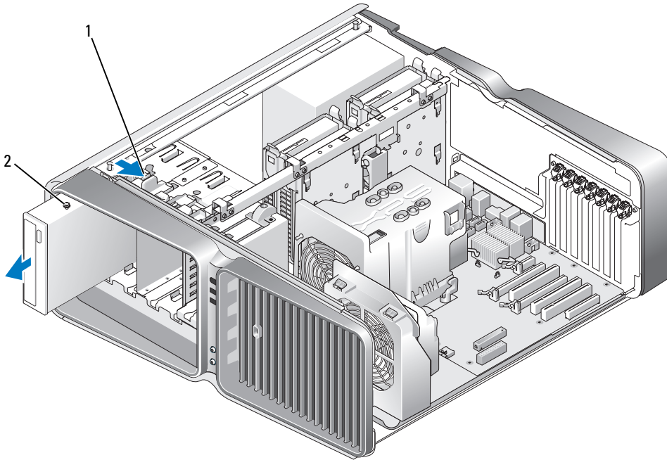
1 Laufwerksperrklinke 2 CD/DVD-Laufwerk
