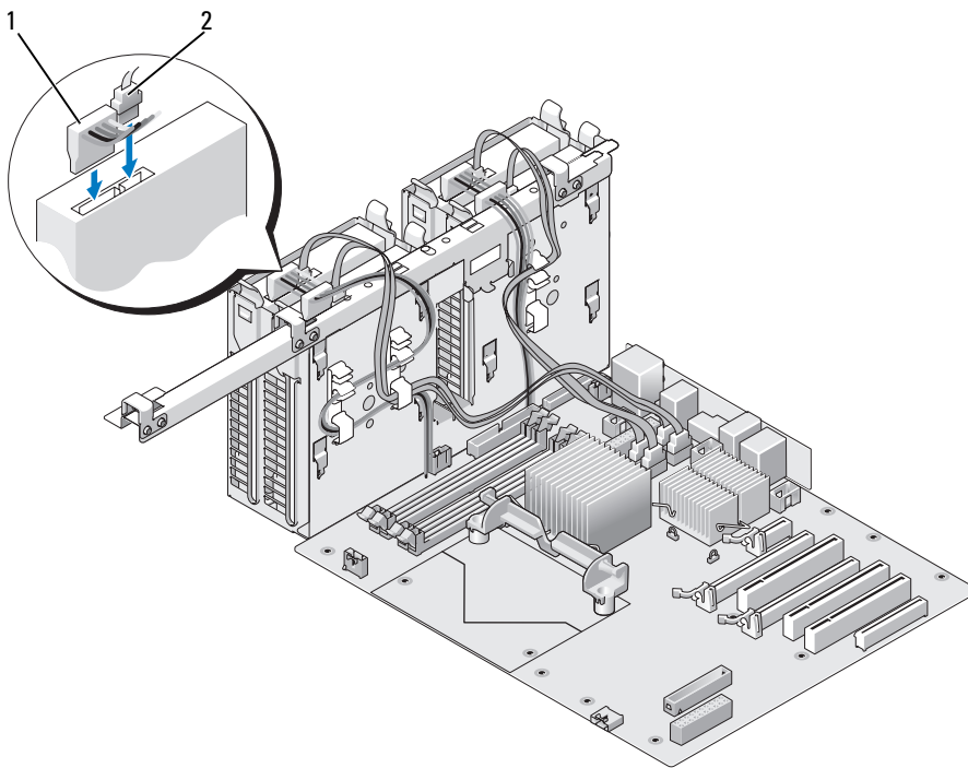
1 Stromversorgungskabel 2 Datenkabel
