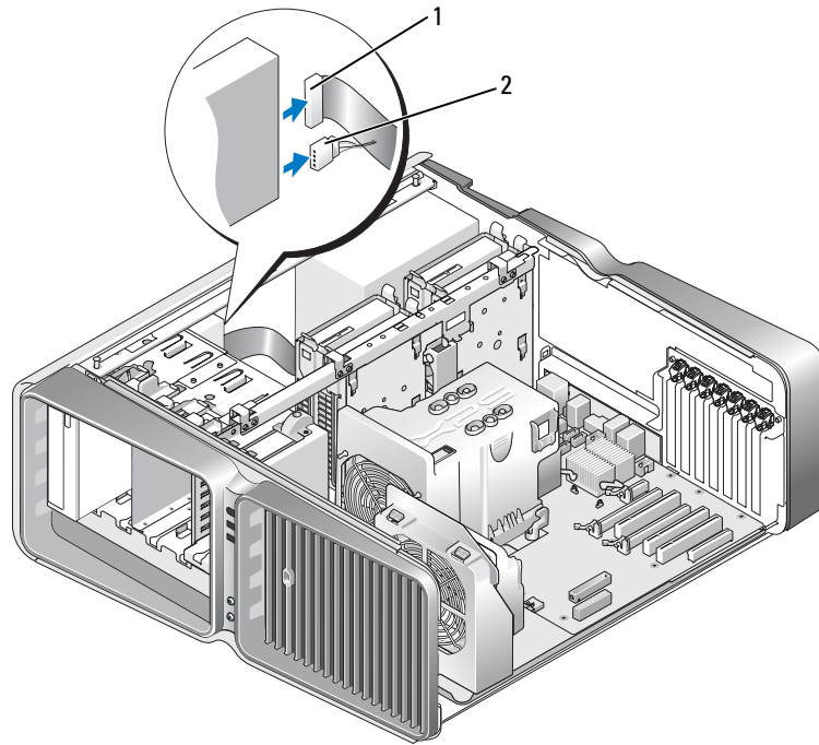
1 Stromversorgungskabel 2 Datenkabel
