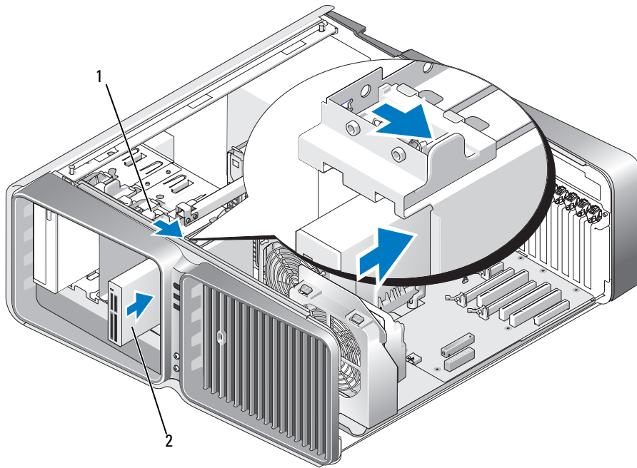
1 Laufwerksperrklinke 2 Medienkartenlesegerät
