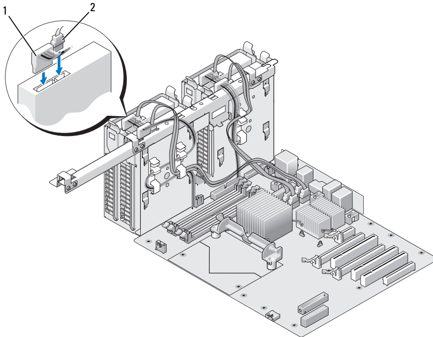
1 Stromversorgungskabel 2 Datenkabel
