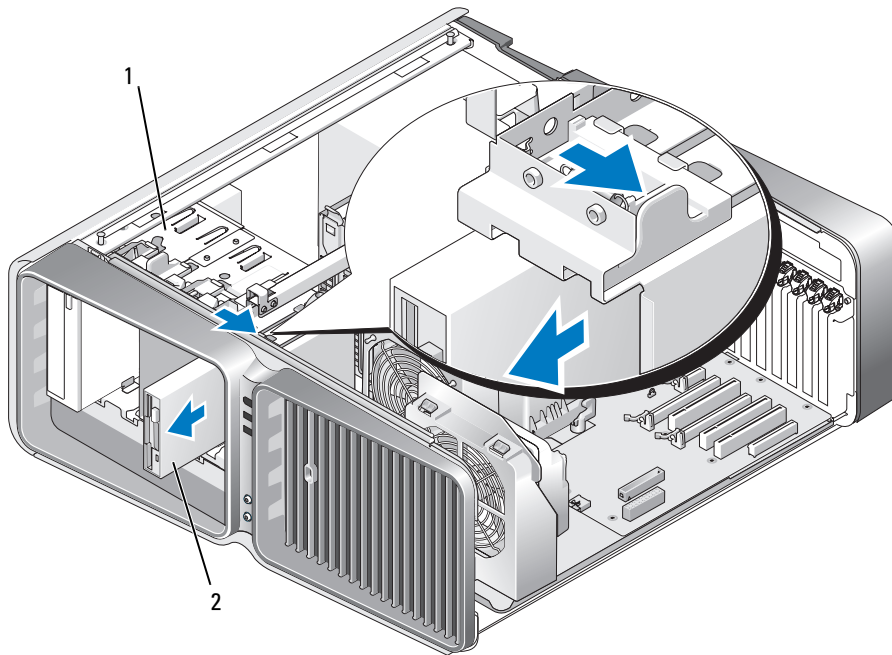
1 Laufwerksperrklinke 2 Diskettenlaufwerk
